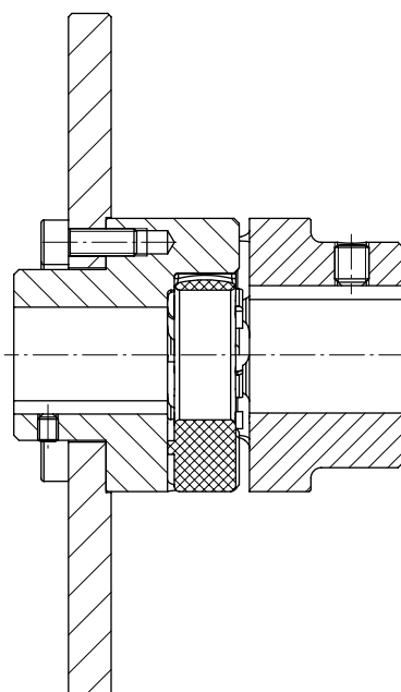
Acoplamientos elásticos de estrella REB ... DCS con disco de freno integrado, forma F
